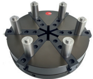
Alu-Stiftbackenfutter Ø = 80, 160, 240 mm
